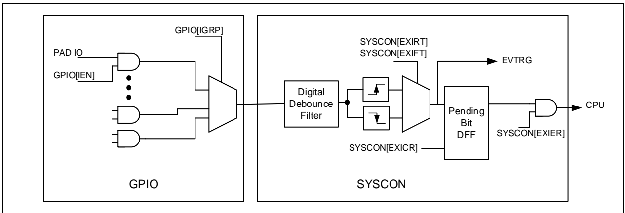
Figure 7-9 外部中断结构示意图
