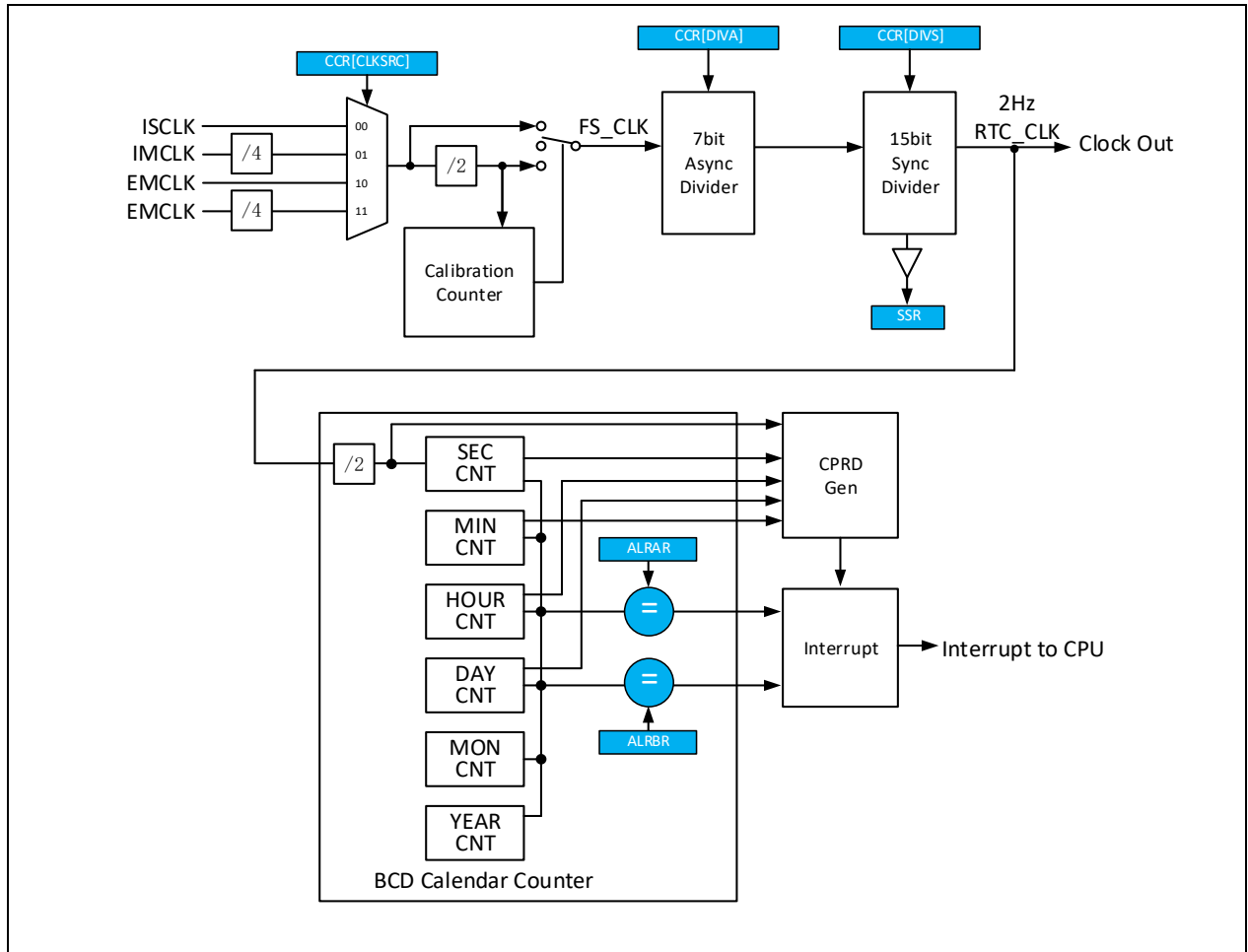
Figure 20-1 功能框图
